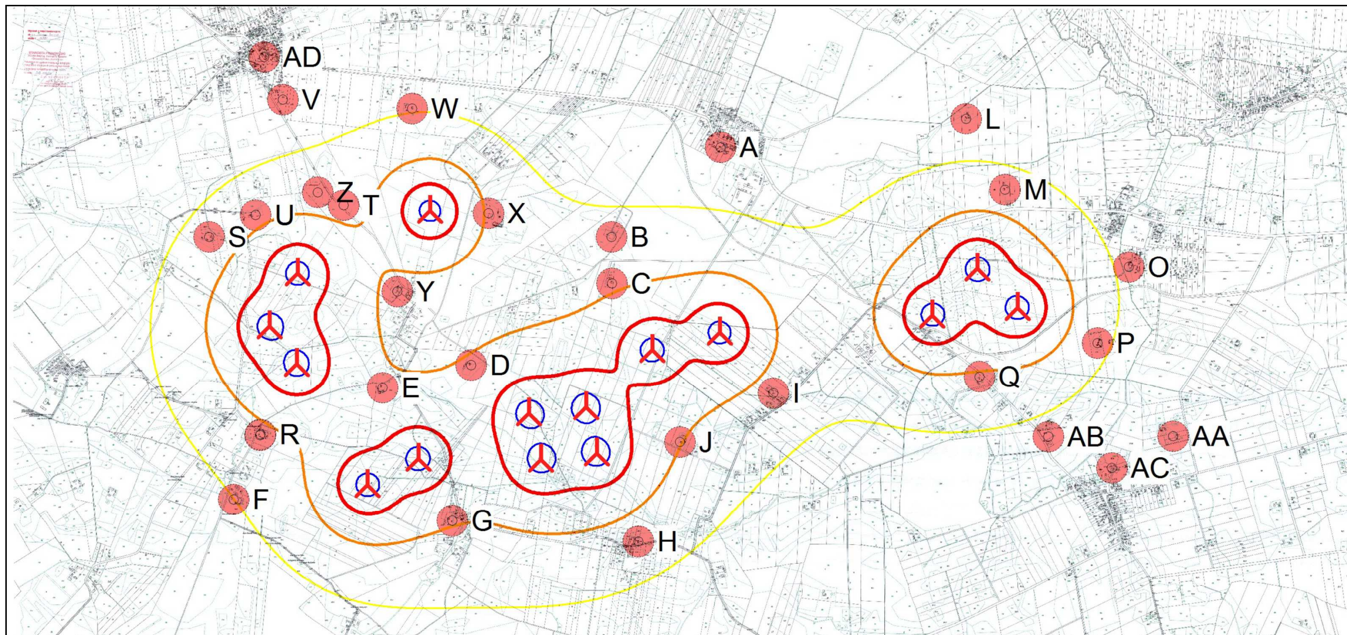
Mapa 2. Rozkład pola akustycznego wokół farmy wiatrowej przedstawiony na mapie ewidencyjnej ( skala 1:5000 - przeskalowana do formatu A3)
