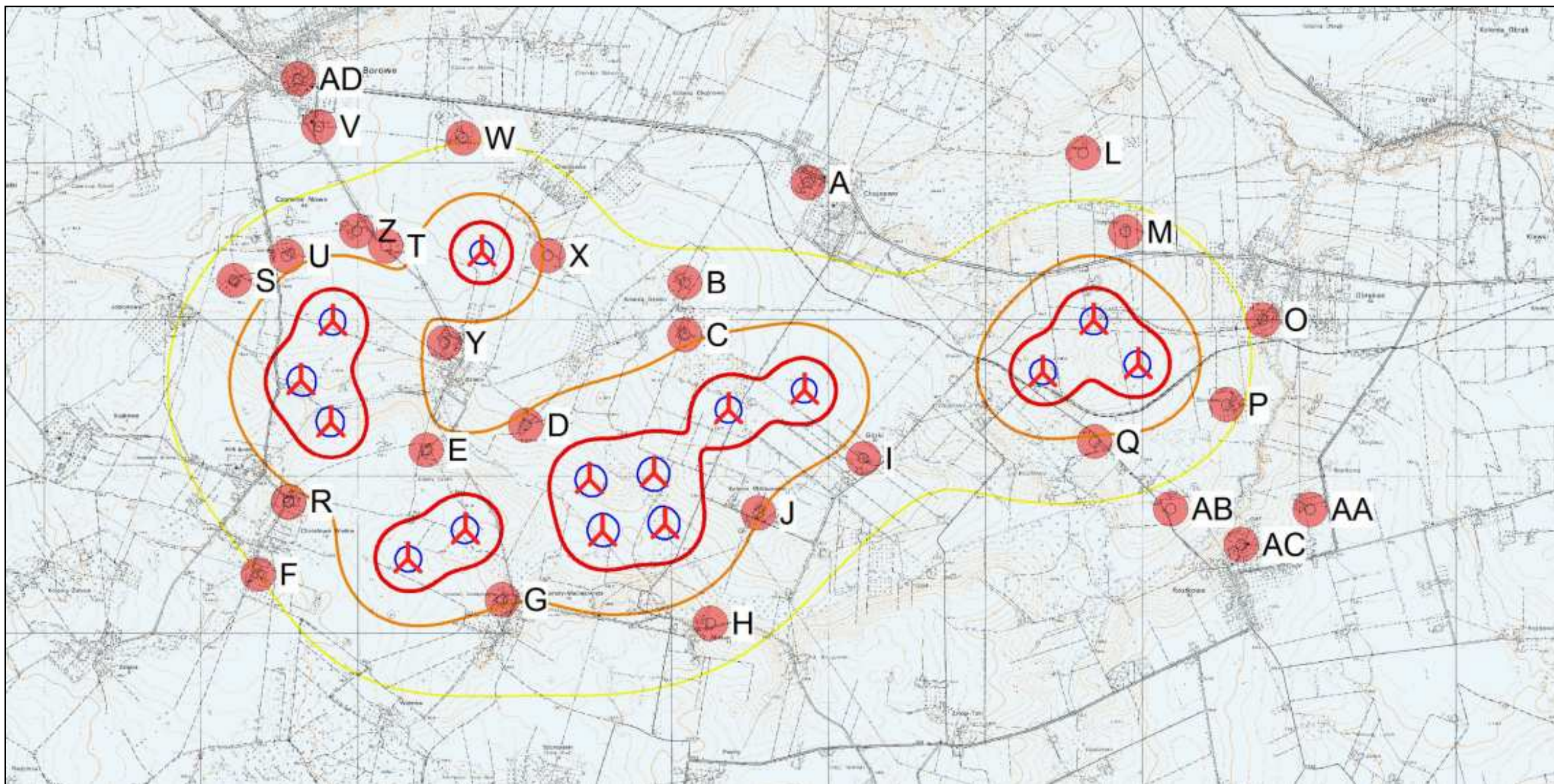
Mapa 1. Rozkład pola akustycznego wokół farmy wiatrowej przedstawiony na mapie topograficznej ( skala 1:10 000 - przeskalowana do formatu A3)
