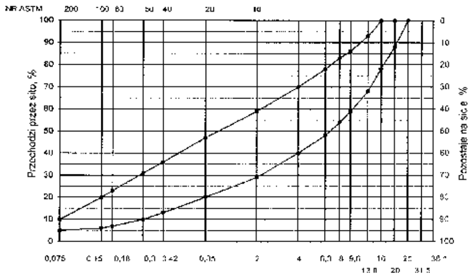
Wymiary oczek sit kwadratowych, mm
